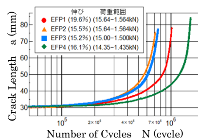
図：同じスラブ材の条件を変えて圧延した鋼板において \sigma_{max}/\sigma_y をそろえた場合の a-N 関係に及ぼす伸び性能の影響
