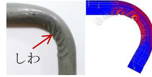
図：引曲げ加工例と曲がり部のひずみ分布
